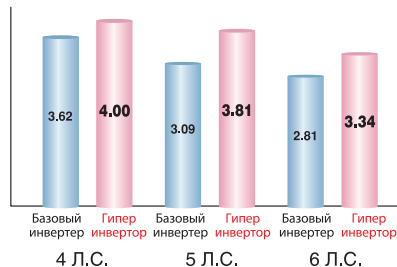
EER (охлаждение)
