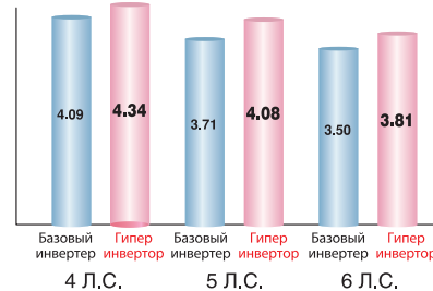
COP (обогрев)
